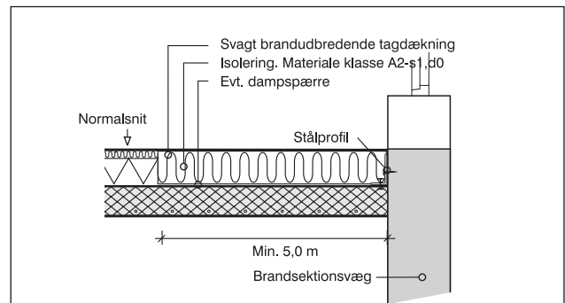
4.3 Spring i bygningshøjde
