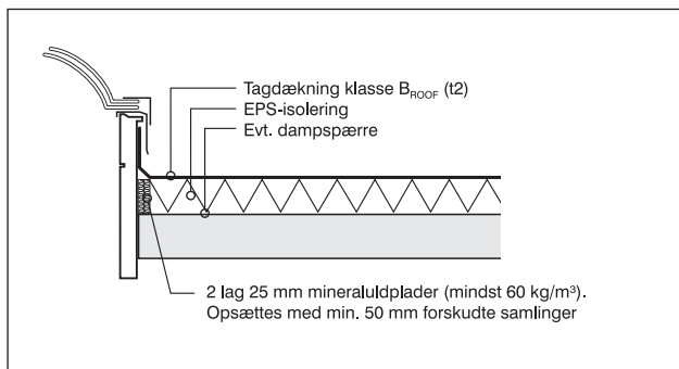
Detalje 3 - Ovenlys
