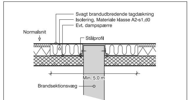
4.2 Brandkammerstatning
