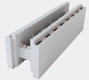
Sundolitt® KUB U19 Rak
